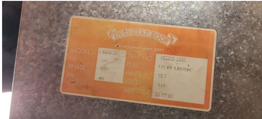
Photo B-1: Existing door operator nameplate (Overhead Door Model RDB-51)
